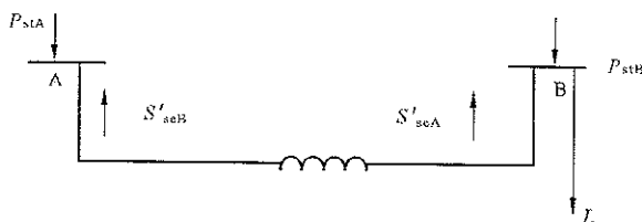
图 2 闪变传递计算示意
